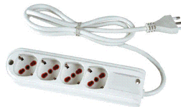
Preso multipla 3 vie universale 10-16 A - 220 V
